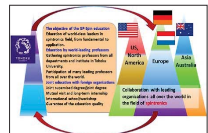
(GP-Spin framework)
