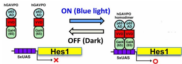
図2：光遺伝学的 Hes1 発現誘導システム
