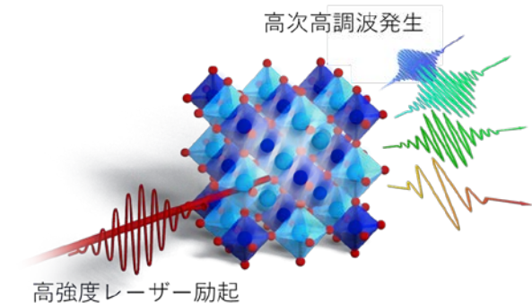
図 2 強電場光パルス照射を固体に照射し、これにより駆動された固体中の電子から放射される高次高調波発生の概念図
