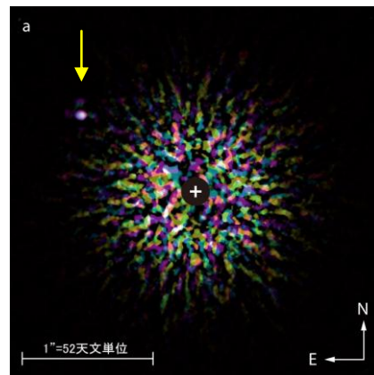
図1 恒星アンドロメダ座κ星のまわりで発見した巨大惑星の赤外線画像。黄色の矢印の先が惑星。
