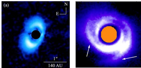
図 2 ギャップ構造および渦巻構造を持つ原始惑星系円盤の近赤外線撮像
