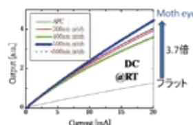
青色LEDの光出力向上
