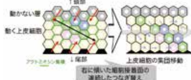
図2 右に傾いた細胞接着面のつなぎ替えが連続して起こることで、上皮細胞を同一方向に集団移動させるしくみの模式図
