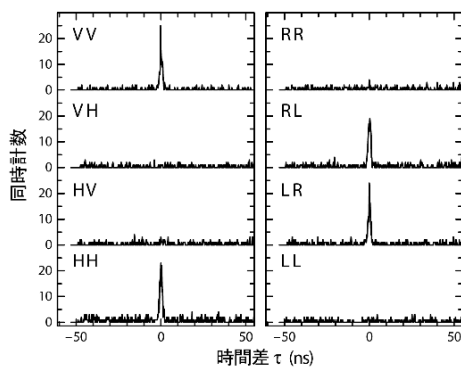
図 1. 半導体(CuCl)から発生した量子もつれ光子の偏光相関の測定例。
