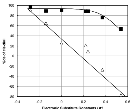
図1. エポキシド水合反応における Hammett 置換基定数とシス選択性の関係 (■: MCM-41 触媒, △: 硫酸触媒)
