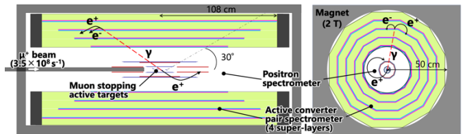
図2 新 \mu \rightarrow e\gamma 探索実験の概念図
