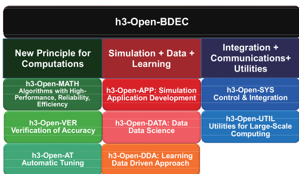
図 1 h3-Open-BDEC の概要
