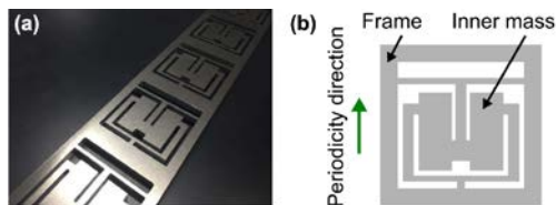
図2 完全バンドギャップをもつ音響メタマテリアル梁(metabeam)の写真(a)と、その単位構造(b)。[2]
