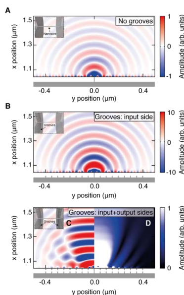
図1 異常音響透過(EAT)のシミュレーションにおいて、3つの構造についてナノワイヤを透過した音場の比較。(A)両側に溝がない場合より、(B)入射側に溝がある場合の方が透過音場が強くなる。さらに(C),(D)出力側にも溝を付けると、音響場が収束する。[1]
