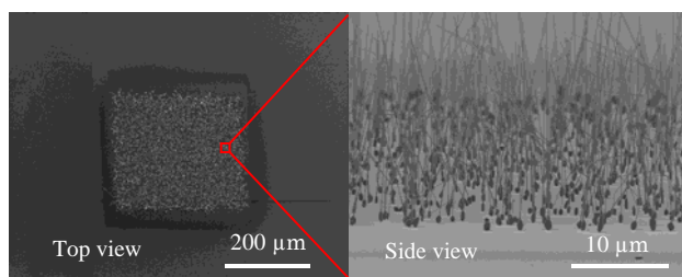
図1 高密度Alナノワイヤ
