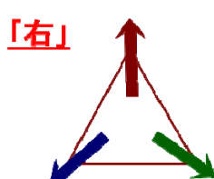
【カイラリティ +】
