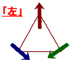
【カイラリティ -】
