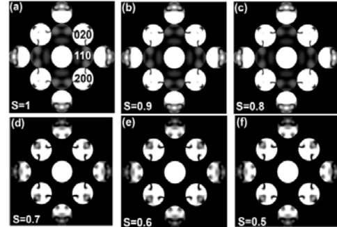
図3 FeNi- L1_0 規則相のシミュレーション模擬NBDパターン (a): S=1 , (b): S=0.9 , (c): S=0.8 , (d): S=0.7 , (e): S=0.6 , (f): S=0.5 超格子反射は、 S \geq 0.8 のときに確認が可能
