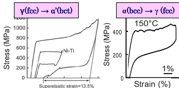
図1 FeNiCoAlTaB および FeMnAlNi 合金の超弾性特性
