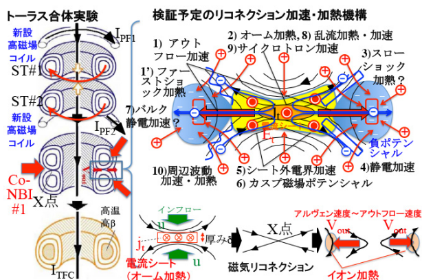
図1 トラスプラズマ合体実験(左)とそれを用いて検証予定の磁気リコネクションの粒子加速・加熱機構(右)
