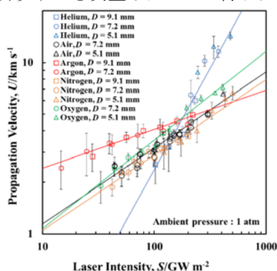
図2 様々なガス種における放電伝播速度のレーザー強度依存性
