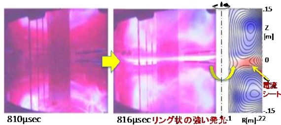
TS-3U の合体過程の光学写真 (左 2 枚, 電流シートの強い発光), 磁気面とトロイダル密度(右)
