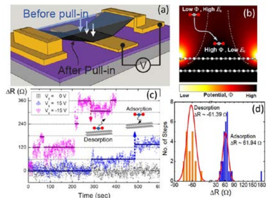
図 1 (a)GNEMS センサー構造, (b)基板電界印加による CO 2 分子閉込めポテンシャル分布, (c)分子吸着・脱離に伴うチャンネル抵抗時間変化, (d)抵抗変化の統計分布 [1]
