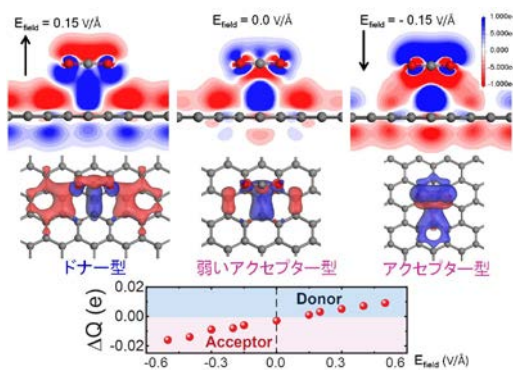
図2 物理吸着したCO 2 分子-グラフェン間電荷移動の電界依存性[2]
