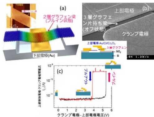
図3 (a) 2層両持ち梁型[4]、および(b) 3層片持ち梁型GNEMSスイッチと、(c) そのスイッチング特性
