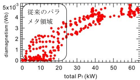
図2：プラズマの平均ベータ値を表わす反磁性磁束（縦軸）とECHパワーの関係。ECHシステム増強と改善によって従来のパラメタ領域から大幅に拡大した。局所ベータ値は1に達したと考えられる。
