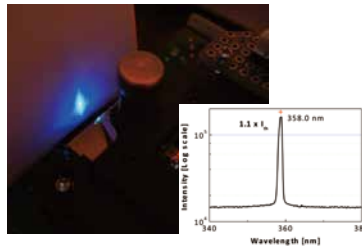
紫外線レーザーダイオード発振の様子
