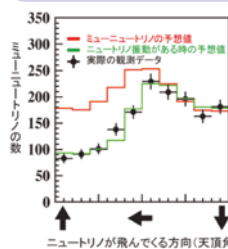
スーパーカミオカンデで観測されたミューニュートリノ
