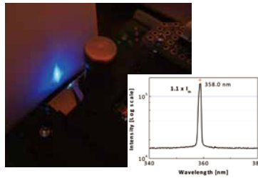
紫外線レーザダイオード発振の様子
