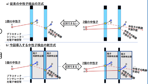
図2 中性子検出方式（従来型：a）、今回開発する新方式 b)
