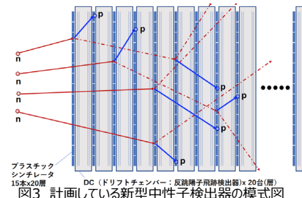
図3 計画している新型中性子検出器の模式図
