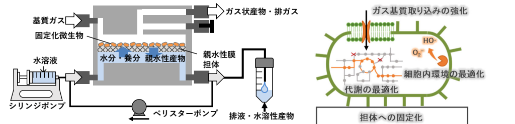
図3 気相微生物反应用リアクターの一例（気液界面型リアクター）
