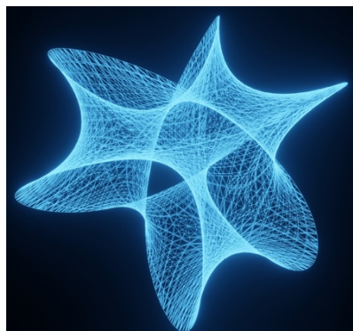
超弦理論に現れる6次元カラビ-ヤウ空間の3次元射影図
