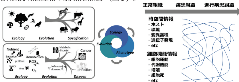
図1 生物学（生態環境-生物進化-種分化）と疾患生物学（微小環境-マイクロ進化-疾患発症・進展）の類似性。環境変化、遺伝子変異、細胞機能などの様々な情報の変化が複雑に絡み合い、疾患が発症・進展する様子を描いた。本研究ではこうした絡み合いを解きほぐし、病気の理解を深める
