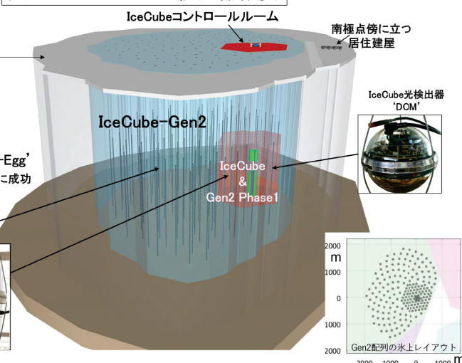
図1: IceCube-Gen2検出器概要
