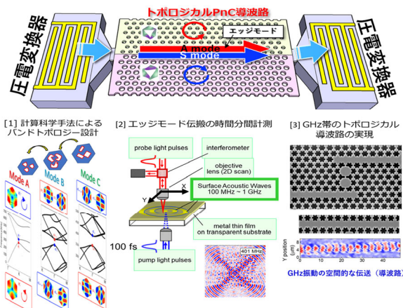
図1 本研究で設計するマルチモードトポロジカルフォノンニックデバイスの模式図(上)と、その[1]設計・[2]可視化・[3]GHz帯実装・高機能化のための各要素技術。
