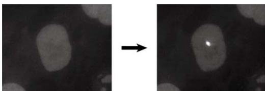
図1 局所紫外線照射部位へのEGFP融合XPCの集積
