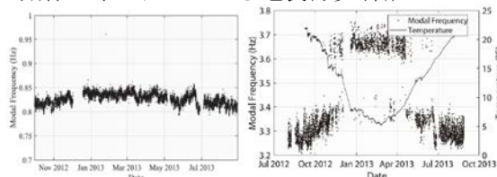
図 2 ギルランディエナの曲げモード(左)とねじれモード(右：アーチの影響)の季節変動
