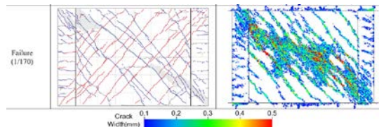
図 1 実験による乾燥下 RC 壁亀裂状況(左)と剛体バネモデルによる亀裂再現(右)
