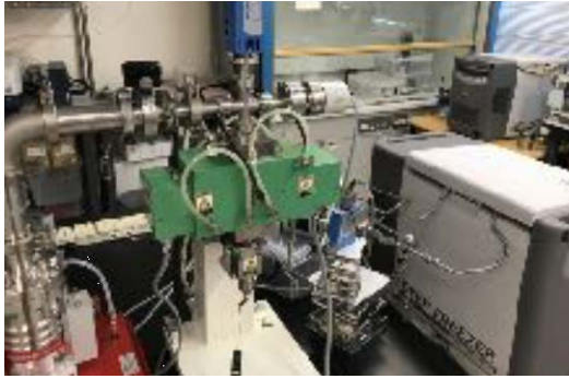
図1 製作した酸素同位体交換実験加熱炉
