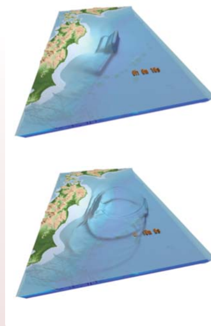
図2 プレートずれ動きモデル(図1)を用いて再現された巨大津波の発生と伝播のようす(地震発生から10秒後(上)、10分後(下))。
