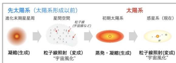
図1 宇宙における固体生成と進化
