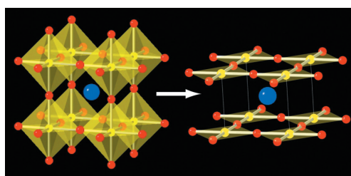
図2 \text{SrFeO}_3 (左)から \text{SrFeO}_2 (右)への反応スキーム。
