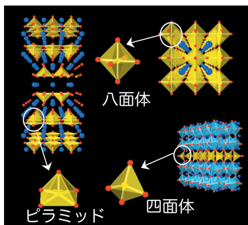
図1 通常の鉄化合物の局所構造。八面体や四面体やピラミッドのような立体的な構造を好みます。鉄原子と酸素原子はそれぞれ黄色、赤色です。
