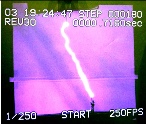
放電(雷)の様子
